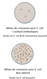
Ratio E. coli BLSE/ E. coli totaux
